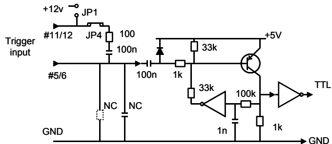
Fig. 5. Trigger input.
