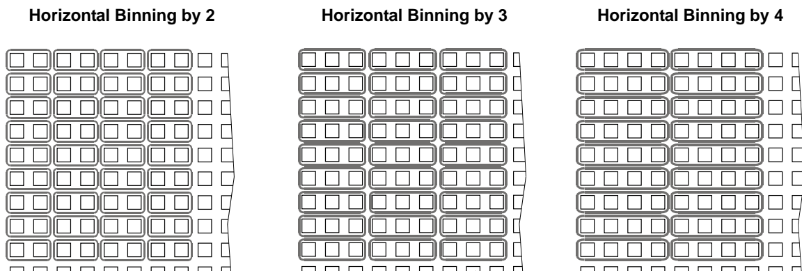
Fig. 81: Horizontal Binning
